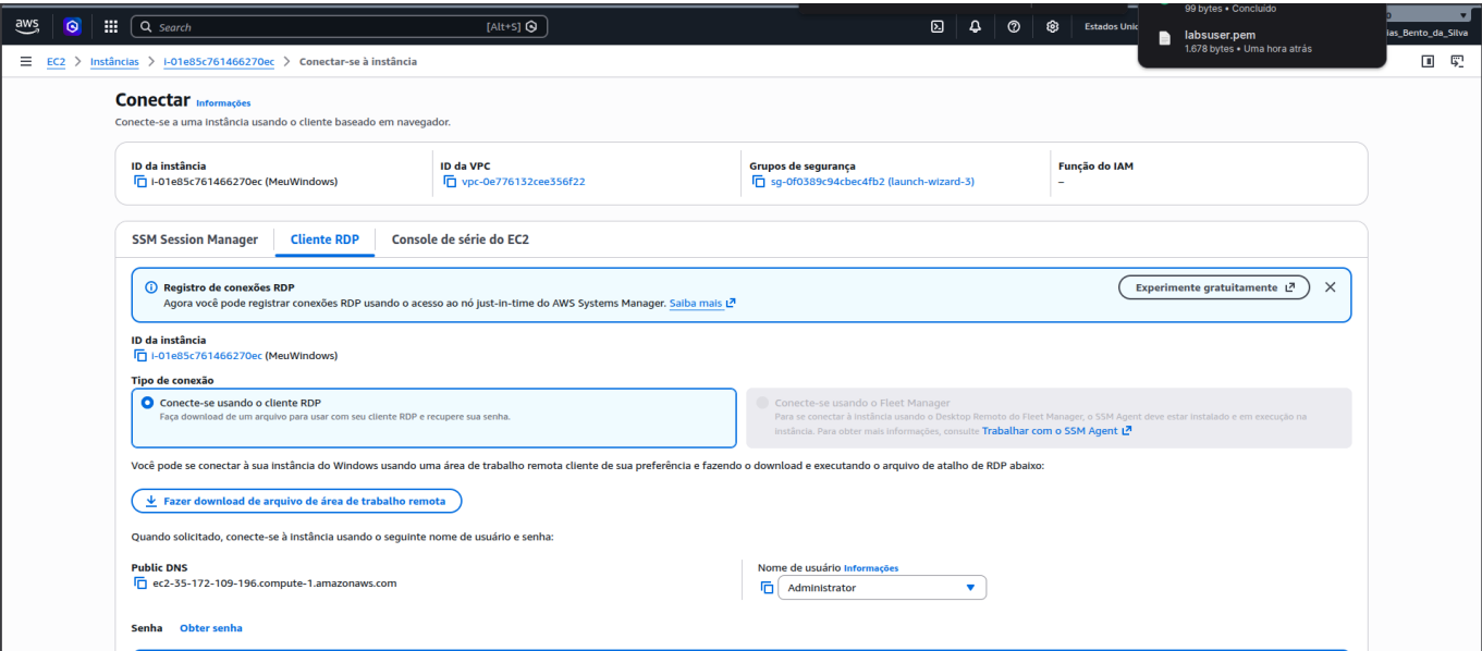
Figura 13: Configuração e download do arquivo RDP para acesso à instância Windows.
